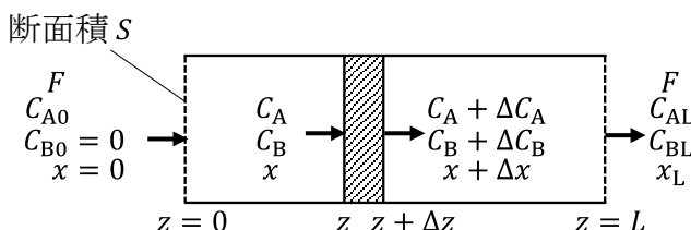
図 5 管型プラグフロー反応器
