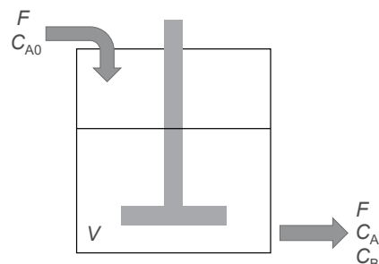
図 1A-2 連続槽型反応器
